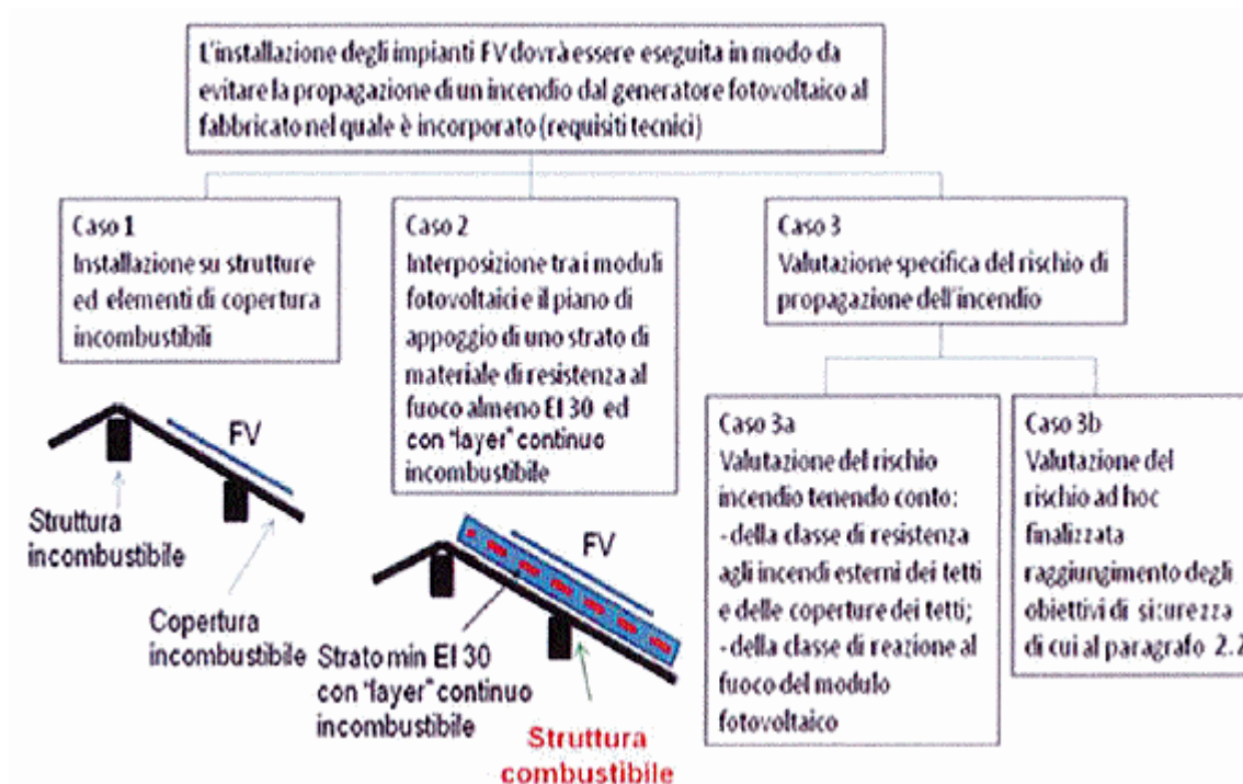
Figura 14 — Modalità di installazione di impianti BAPV
